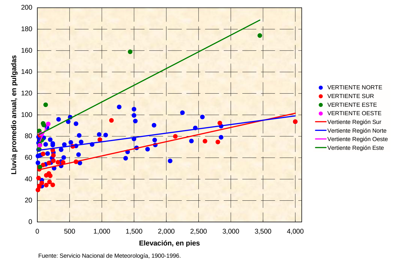
Figura 2-5. Efecto orográfico, lluvia promedio por vertientes de las cordilleras en Puerto Rico.
