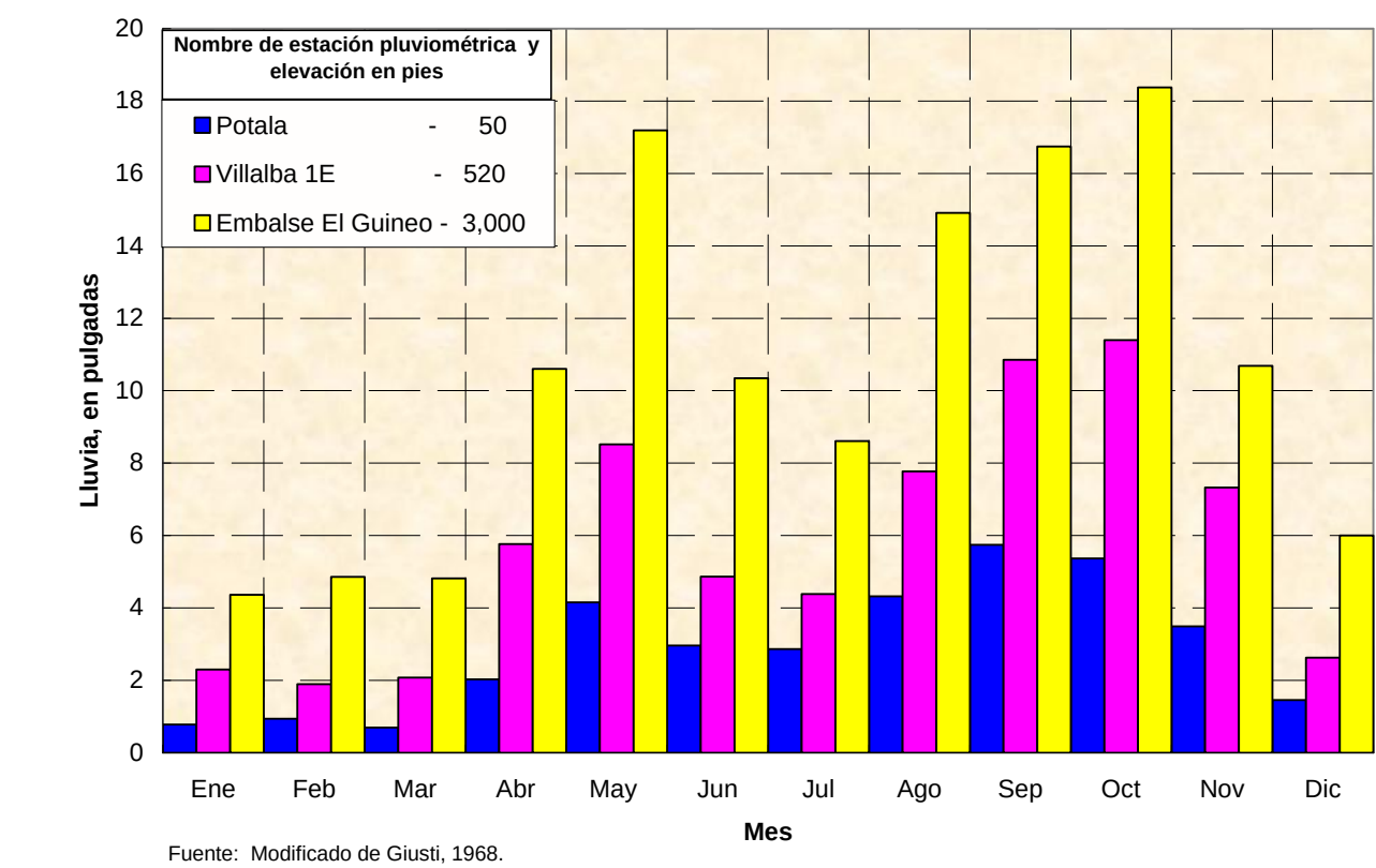
Figura 2-4. Variación en precipitación con la elevación en Puerto Rico.
