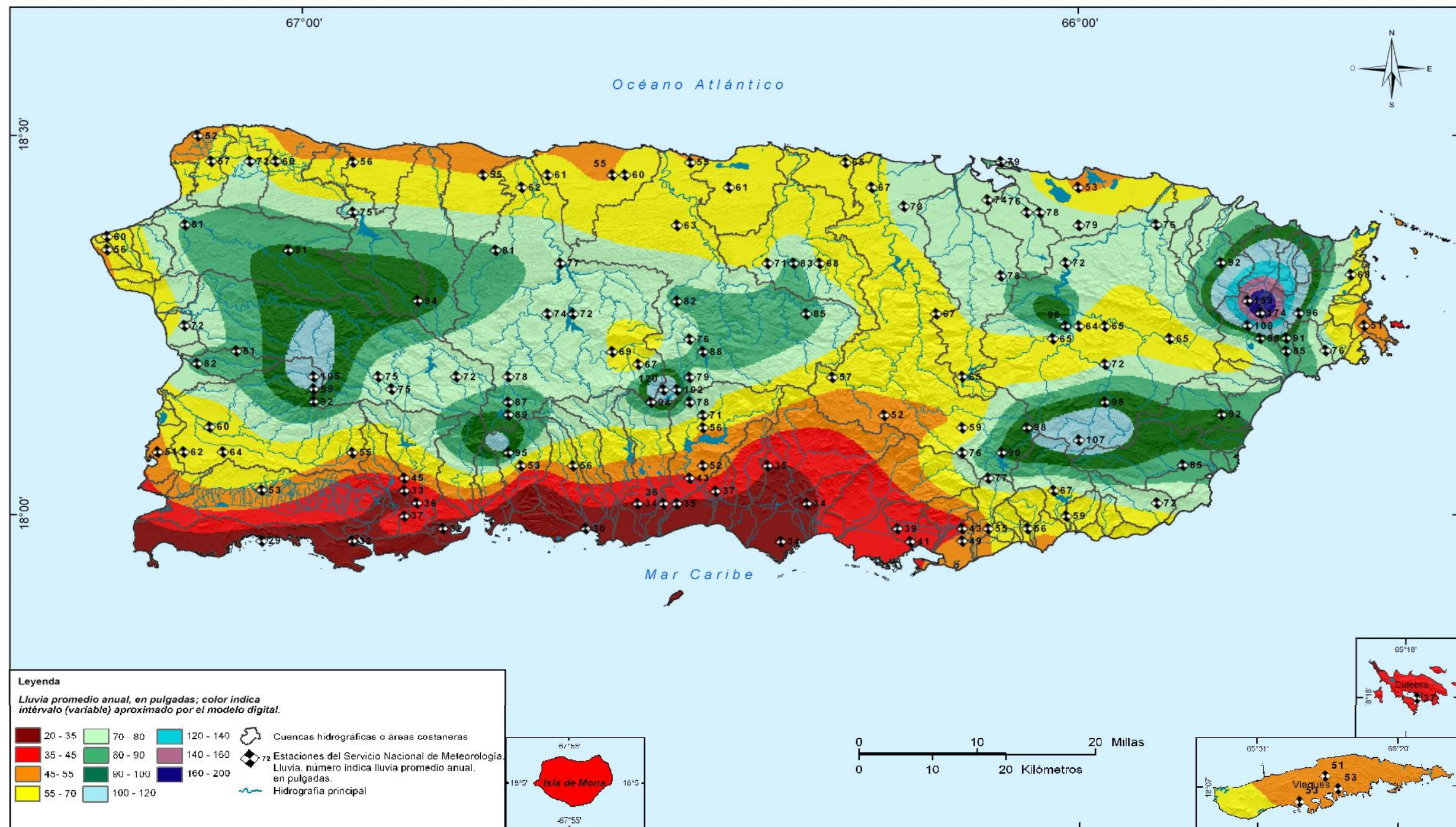
Figura 2-6. Distribución de lluvia promedio en Puerto Rico (datos 1950-1980).
