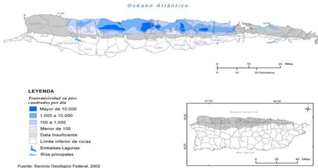
Figura 2. Productividad del Acuífero Superior de la Región del Karso (expresadas como Transmisividad en metros cuadrados por día, que es la unidad utilizada para medir productividad de un acuífero) (Renken, 2002).
