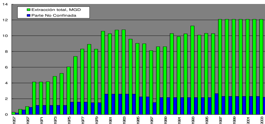
Figura 4. Extracción total, incluyendo estimado de perdidas en camisillas de pozos hincados en la parte confinada del Acuífero Inferior de la Región del Karso de Puerto Rico (USGS, unpublished data).
